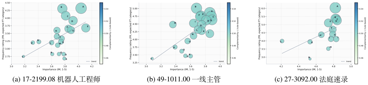
图 4: 三职业任务 DNA 权重分布（IM-FR 散点图），点面积与 w_j 成正比。任务文本图例见附录 B。
