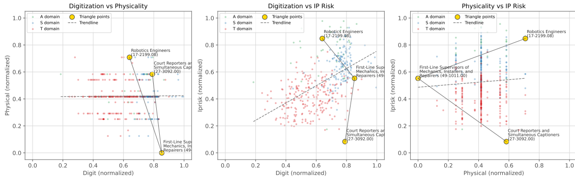
图 2: 全体职业异质性空间的二维投影与最优三点标注（二维面积公式见附录 A.2）
