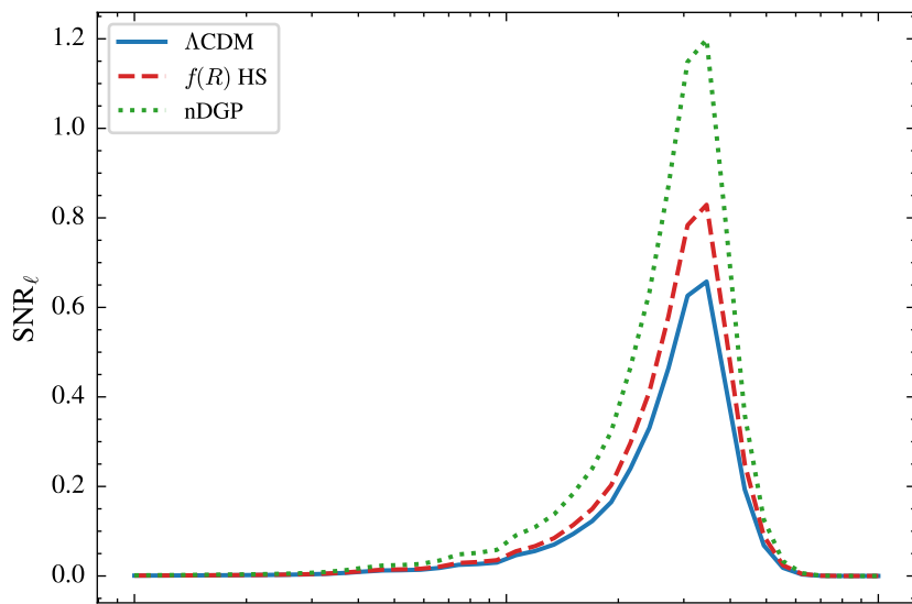
LSST \times Planck
