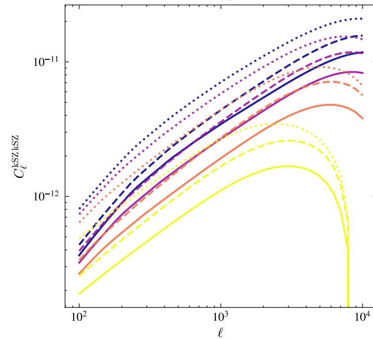
kSZ auto-spectrum
