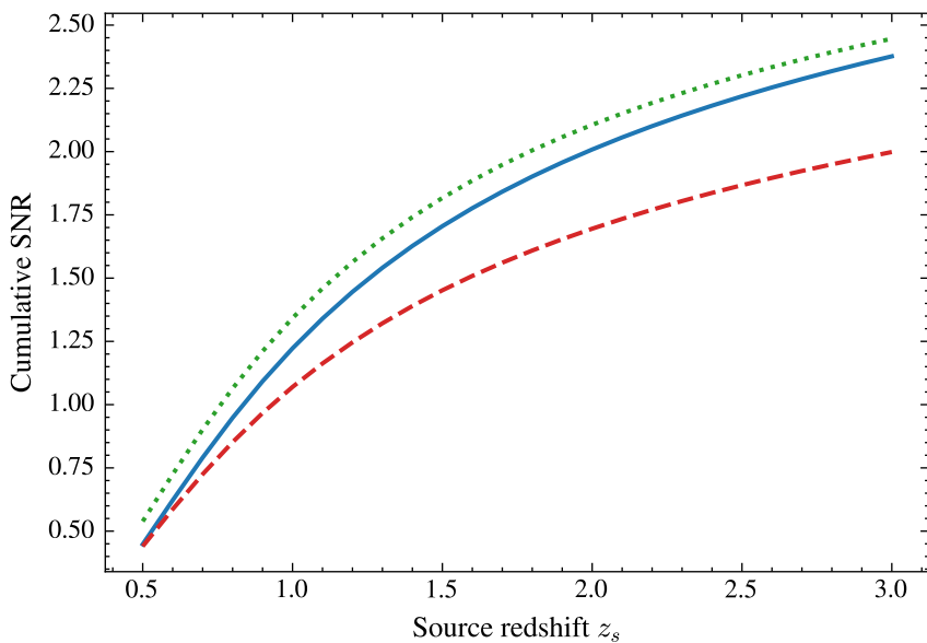
LSST \times Planck
