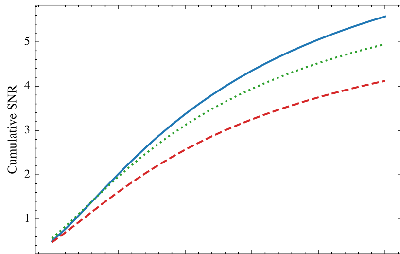
LSST \times SO
