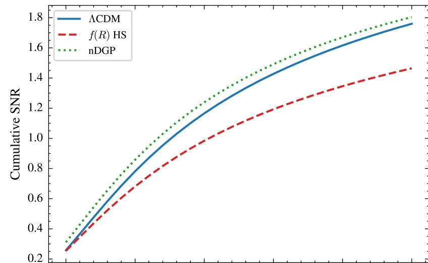
LSST \times Planck
