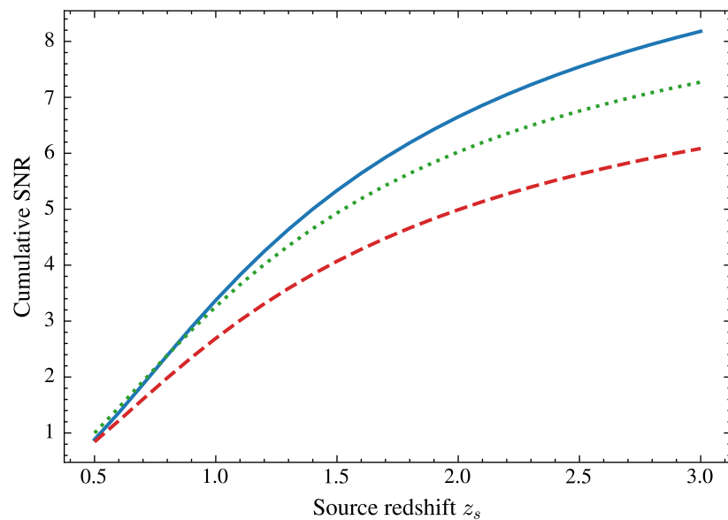
LSST \times SO
