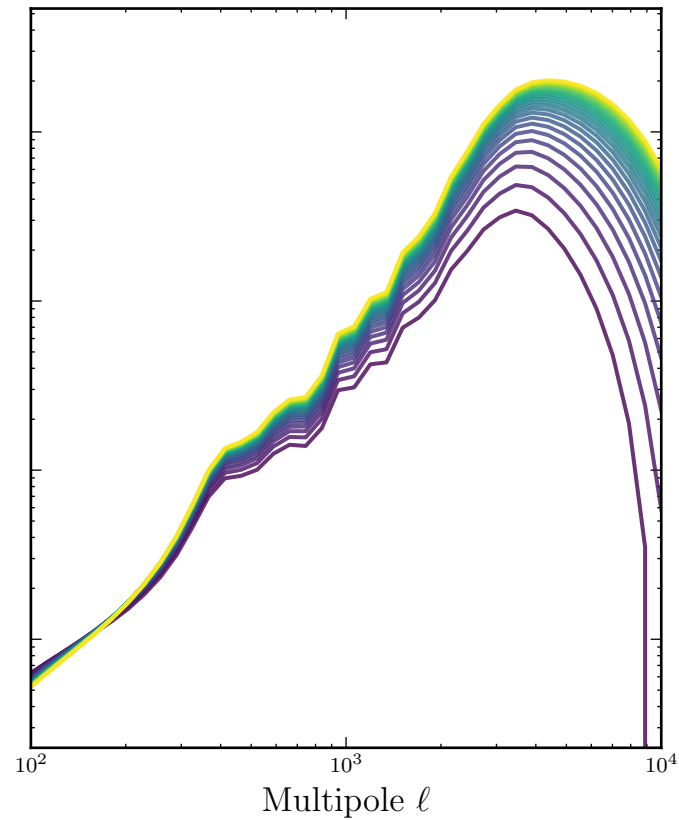
nDGP SNR
