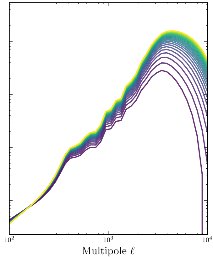
f(R) Hu-Sawicki SNR
