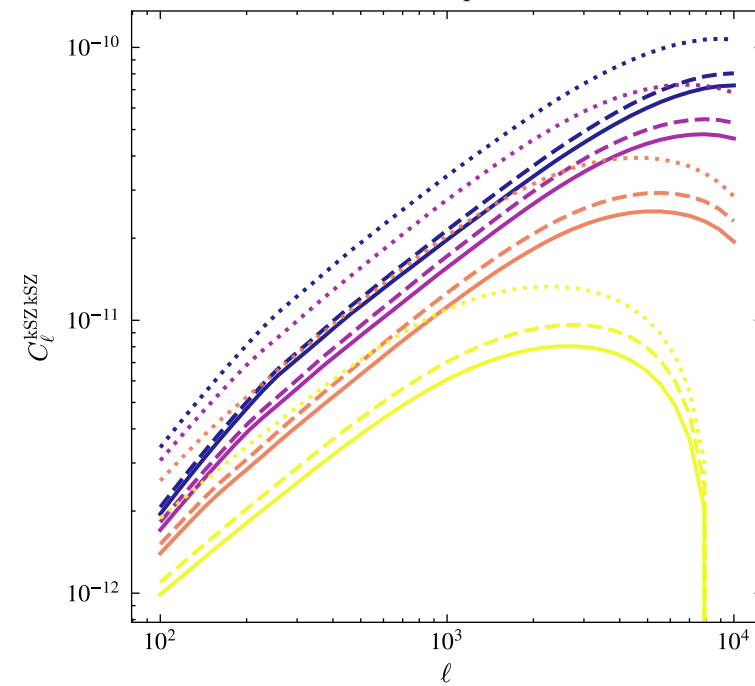
kSZ auto-spectrum
