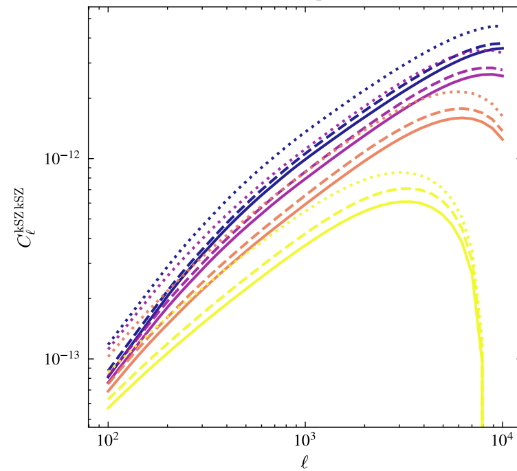
kSZ auto-spectrum
