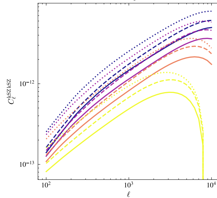
kSZ auto-spectrum
