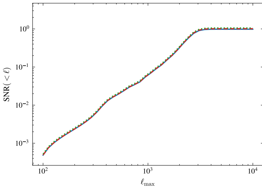
LSST \times Planck
