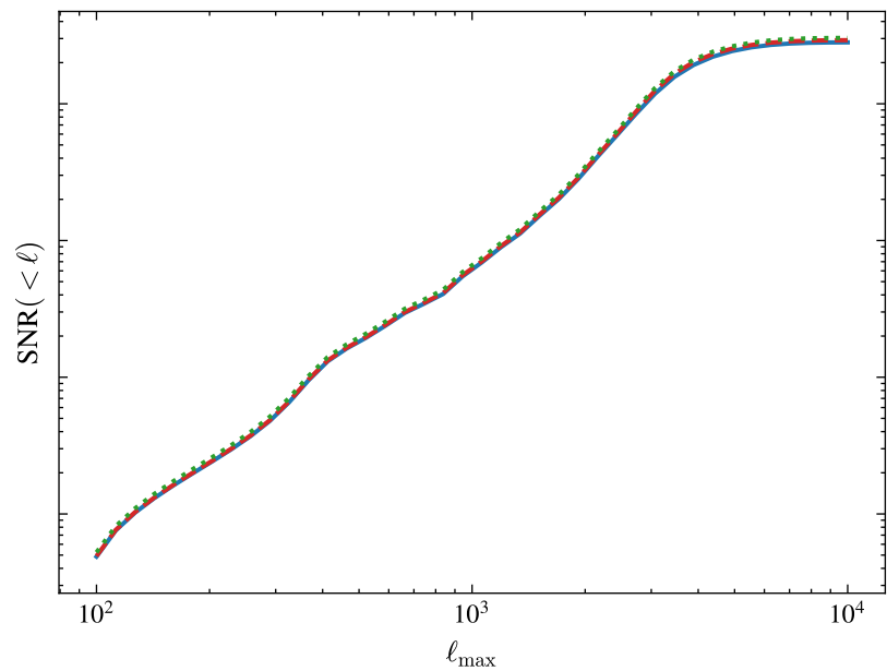
LSST \times SO
