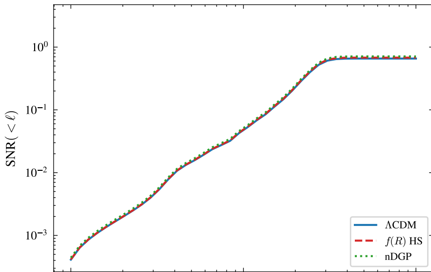
LSST \times Planck
