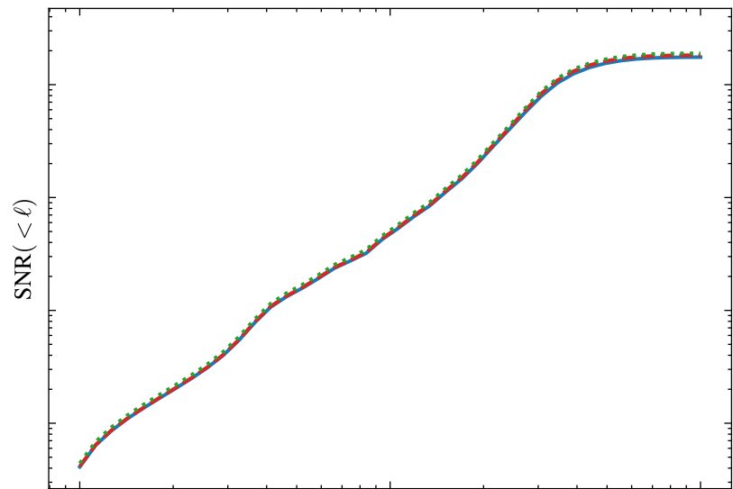
LSST \times SO
