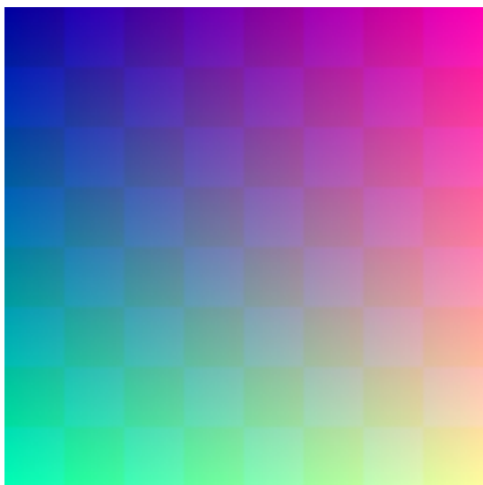
JPEG (DCTDecode):
