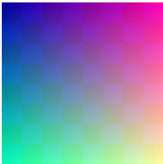
JPEG 2000 (JPXDecode):
