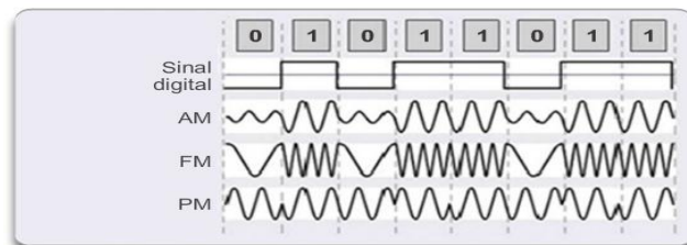
Sinais de Microondas - Sem fio
