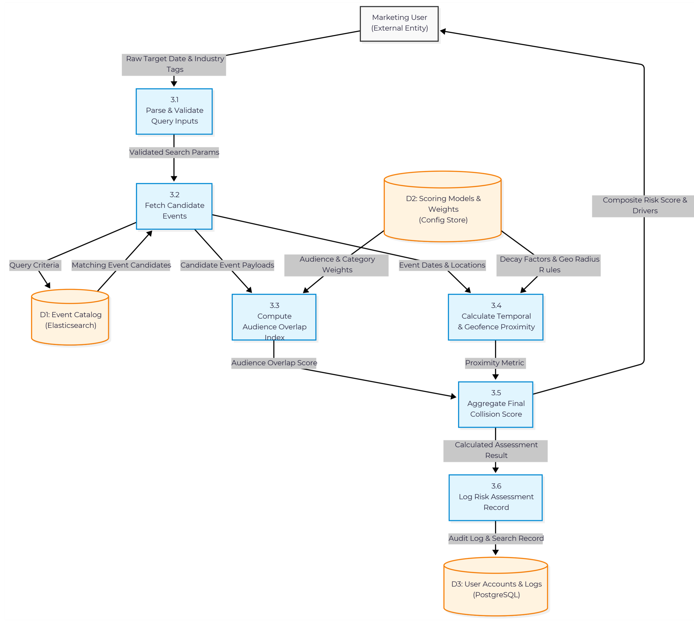
Level-2 DFD
