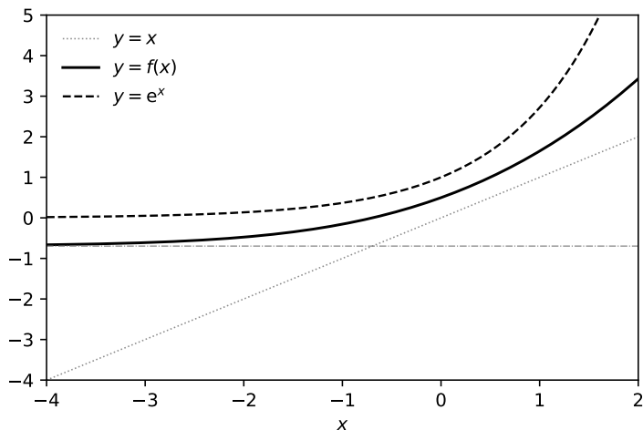
图 1.1: Kneser 的半指数函数 f (实线)、 e^x (虚线) 与对角线。点划线是水平渐近线 y = -0.69602\dots 。脚本 figures/fig1_halfexp.py 。
