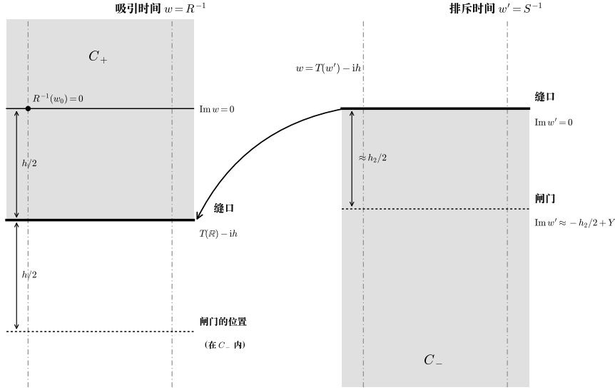
图 5.1: 缝合的两个半柱面 (示意图, 不按比例; figures/fig5_cylinders.py )。左: 吸引时间 w = R^{-1} , 上半柱面 C_+ = \{\text{Im } w \geq -h/2\}/\mathbb{Z} 。右: 排斥时间 w' = S^{-1} , 下半柱面 C_- = \{\text{Im } w' \leq 0\}/\mathbb{Z} 。右侧缝口上的点 w' 粘到左侧的 T(w') - ih 。闸门 (第 7 章中 T 收敛到逆 horn 映射的地方) 在排斥时间里位于缝口下方约 h_2/2 处; 换到吸引时间, 它在缝口下方约 h/2 、实轴下方约 h 处。
