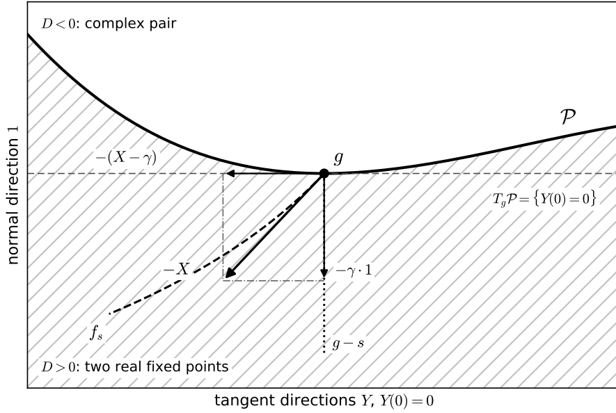
图 9.1: g 附近映射空间的示意图。横轴代表切方向 T_g \mathcal{P} = \{Y(0) = 0\} , 纵轴代表常数方向 1。粗实线是抛物层 \mathcal{P} ; 阴影区 D > 0 是有两个实不动点的实映射, 上方 D < 0 是有一对复共轭不动点的映射。虚线是开折 f_s = g - sX + O(s^2) , 其速度 -X 分解为法向分量 -\gamma \cdot 1 与切向分量 -(X - \gamma) 。点线是平移开折 g - s 。(脚本 figures/fig9_stratum.py )
