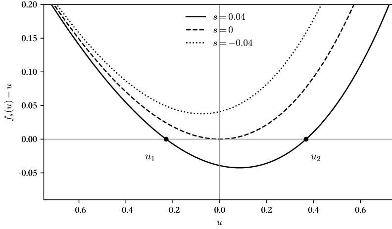
图 4.1: tetration 开折的 f_s(u) - u , f_s(u) = e^{-s+(1-s)u} - 1 (figures/fig4_unfolding.py)。 s = 0.04 : 两个实零点 u_1 = -0.2283, u_2 = 0.3683 (Glutsyuk 一侧); s = 0 : 二重零点; s = -0.04 : 没有实零点 (Lavaurs 一侧)。
