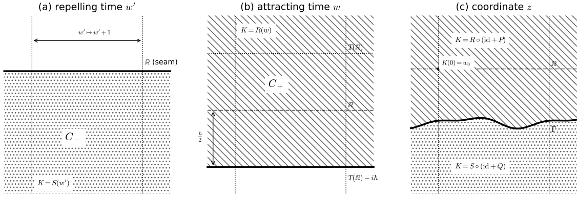
图 6.1: 缝合解的焊接示意 (脚本 figures/fig6_welding.py )。 (a) 排斥时间 w' 中的下半柱面 C_- , 缝是实轴; (b) 吸引时间 w 中的上半柱面 C_+ , 缝是直线 \text{Im } w = -h/2 , 它是 \mathbb{R} 在 T - ih 下的像; 点线 T(\mathbb{R}) 在实轴上方半个周期处。 (c) 单值化坐标 z : 缝 \Gamma 是 \text{Im } z \approx -h/2 附近的一条曲线, 上方 K = R \circ (\text{id} + P) , 下方 K = S \circ (\text{id} + Q) , K(0) = w_0 。虚线是基本域的边界。
