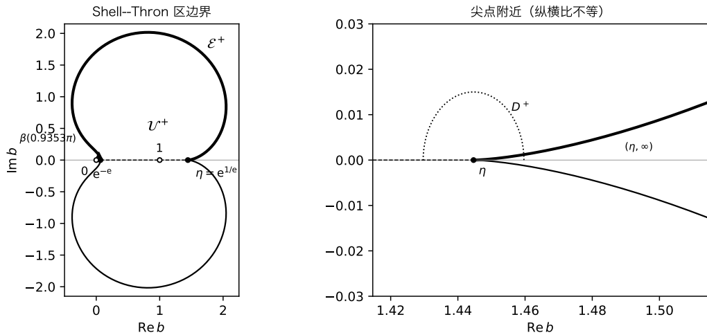
图 10.1: Shell–Thron 区的边界 \beta(\alpha) (粗线为上中性弧 0 < \alpha < \pi ), 实段 [e^{-e}, \eta] (虚线), 奇点 0、1 (空心点), 以及 定理 10.20 中的 \beta(0.9353\pi) 。右图放大尖点 \eta 附近, 外侧实射线 (\eta, \infty) 夹在两条边界弧形成的细角中, 虚线半圆是 定理 10.12 中的 D^+ 。脚本 figures/fig10_shell_thron.py 。
