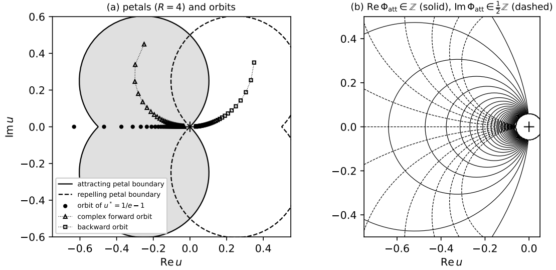
图 3.1: g(u) = e^u - 1 . (a) 吸引花瓣（灰色，实线边界）与排斥花瓣（虚线边界），取示意值 R = 4 ( \zeta = -2/u )；实心点是 u^* = 1/e - 1 的实轨道，三角是一条复轨道，二者沿负实轴切向趋于 0；方块是一条后向轨道，沿正实轴趋于 0。(b) \Phi_{\text{att}} 的坐标网：实线 \text{Re } \Phi_{\text{att}} \in \mathbb{Z} ，虚线 \text{Im } \Phi_{\text{att}} \in \frac{1}{2}\mathbb{Z} ；相邻两条实线之间是 g 的一个基本域。脚本 figures/fig3_petals.py 。
