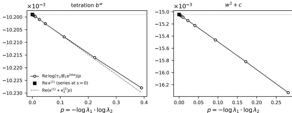
图 8.1: \text{Re} \log(\tau_1/B_1 e^{2\pi i a})/p 随 p 的变化 (圆圈, 双曲侧直接计算, \lambda_1 = 0.5, \dots, 0.98 ), 方块为 s=0 处级数给出的 \text{Re} \kappa^{(1)} 。左: tetration, 虚线为 \text{Re}(\kappa^{(1)} + \kappa_2^{(1)}p) ; 右: 二次族 w^2 + c 。数值。
