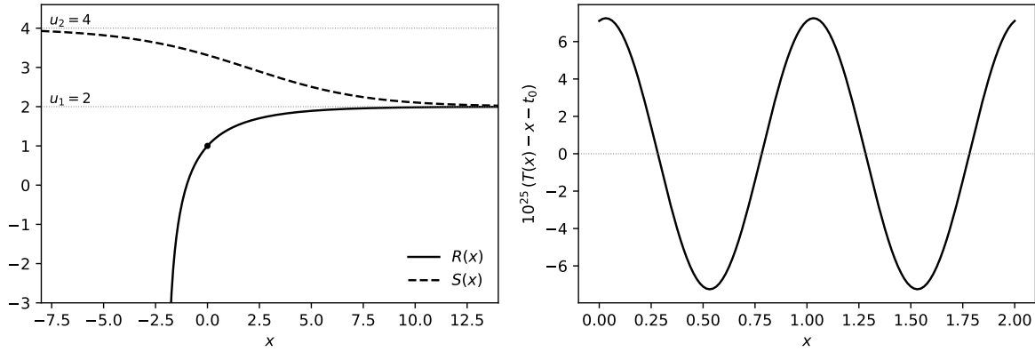
图 2.1: b = \sqrt{2} 。左: R(x) (实线, x > -2 ) 与 S(x) (虚线), 点为 R(0) = 1 , 点线为不动点 2、4。右: 转移映射的非常数部分 10^{25}(T(x) - x - t_0) , 它是实值、1-周期的, 振幅 2|t_1| = 7.25 \times 10^{-25} (例 2.22)。脚本 figures/fig2_regular.py 。
