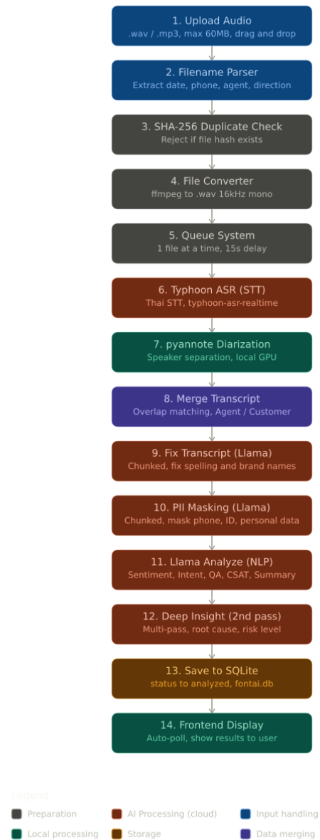
ภาพที่ 3.2 Workflow Diagram (Typhoon Pipeline)
