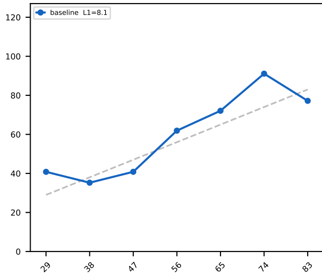
Baseline
