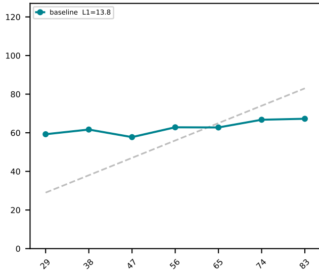
Gemini Flash
