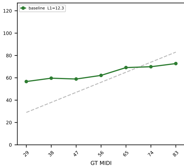
GPT-4o
