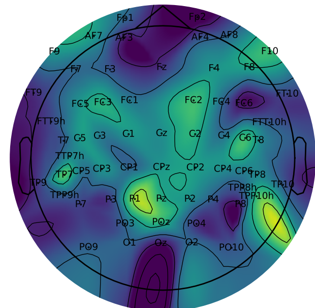
PhysionetMI (n=64)
