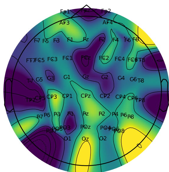
Weibo2014_8.2s (n=60)
