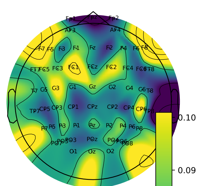
Weibo2014_4.2s (n=60)
