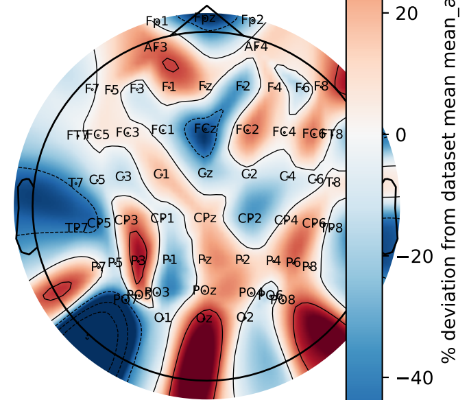
Weibo2014_4.2s (n=60)
