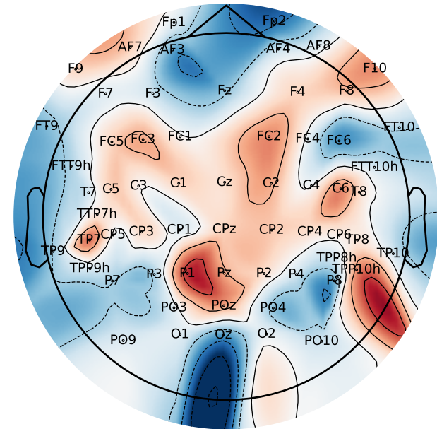
PhysionetMI (n=64)
