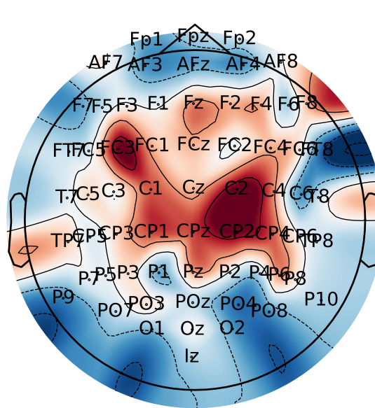
Cho2017 (n=64)
