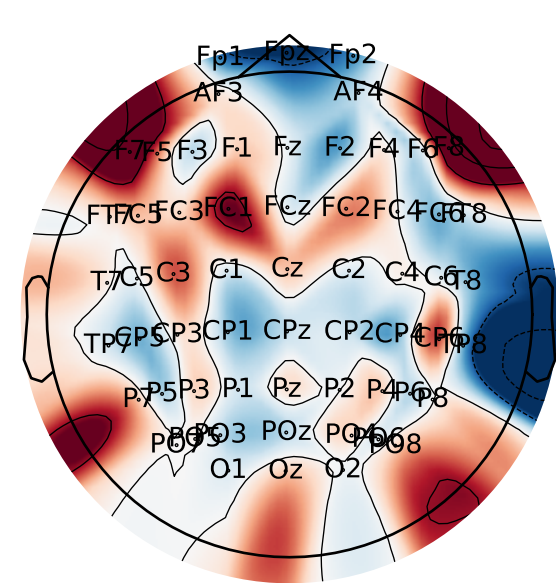
Stieger2021 (n=60)
