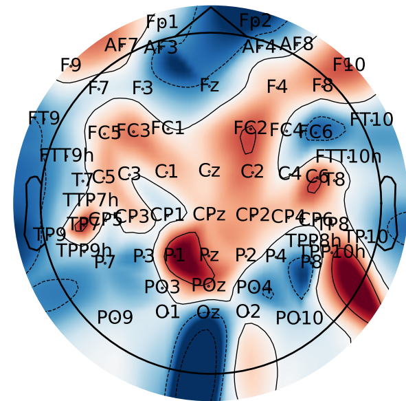
Lee2019_MI (n=62)
