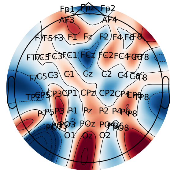
Weibo2014_4.2s (n=60)
