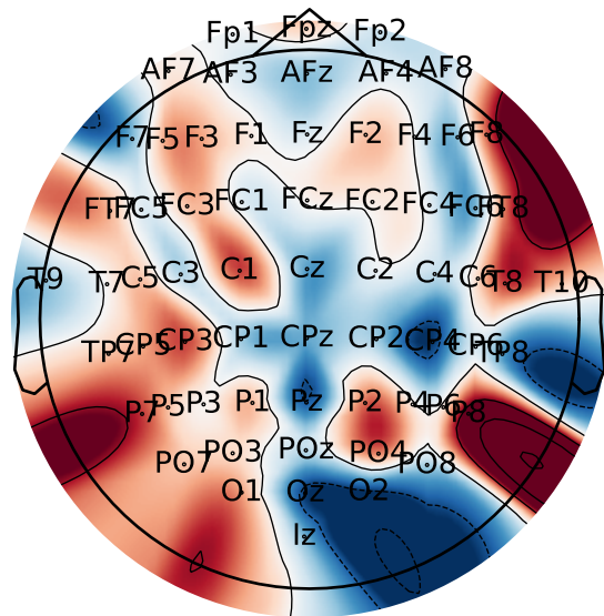
Weibo2014_8.2s (n=60)
