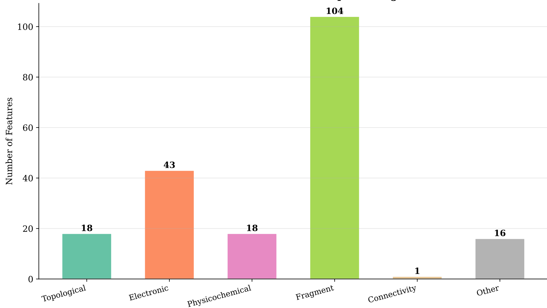
Stokes et al.: 200 RDKit Descriptor Categories
