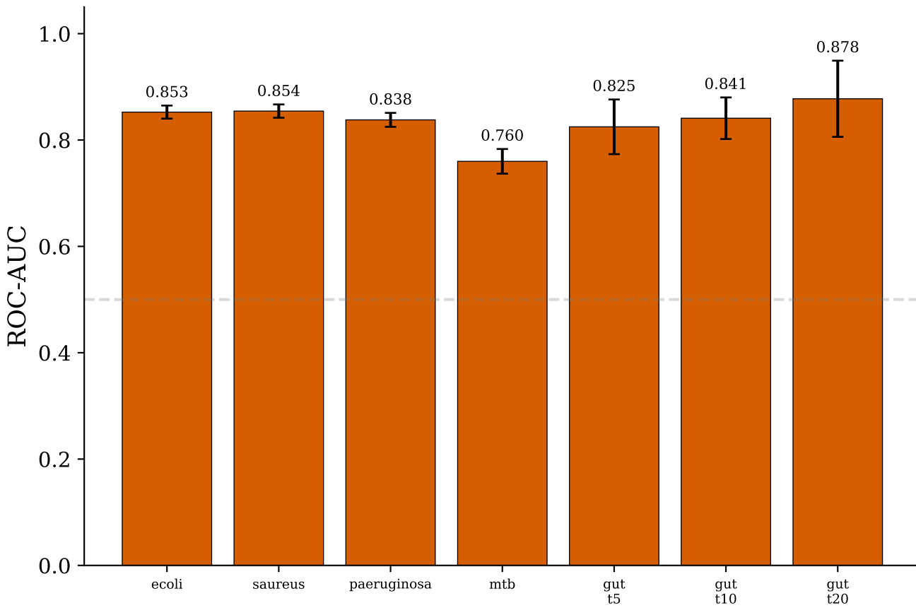
A. D-MPNN ROC-AUC (5-fold scaffold CV)
