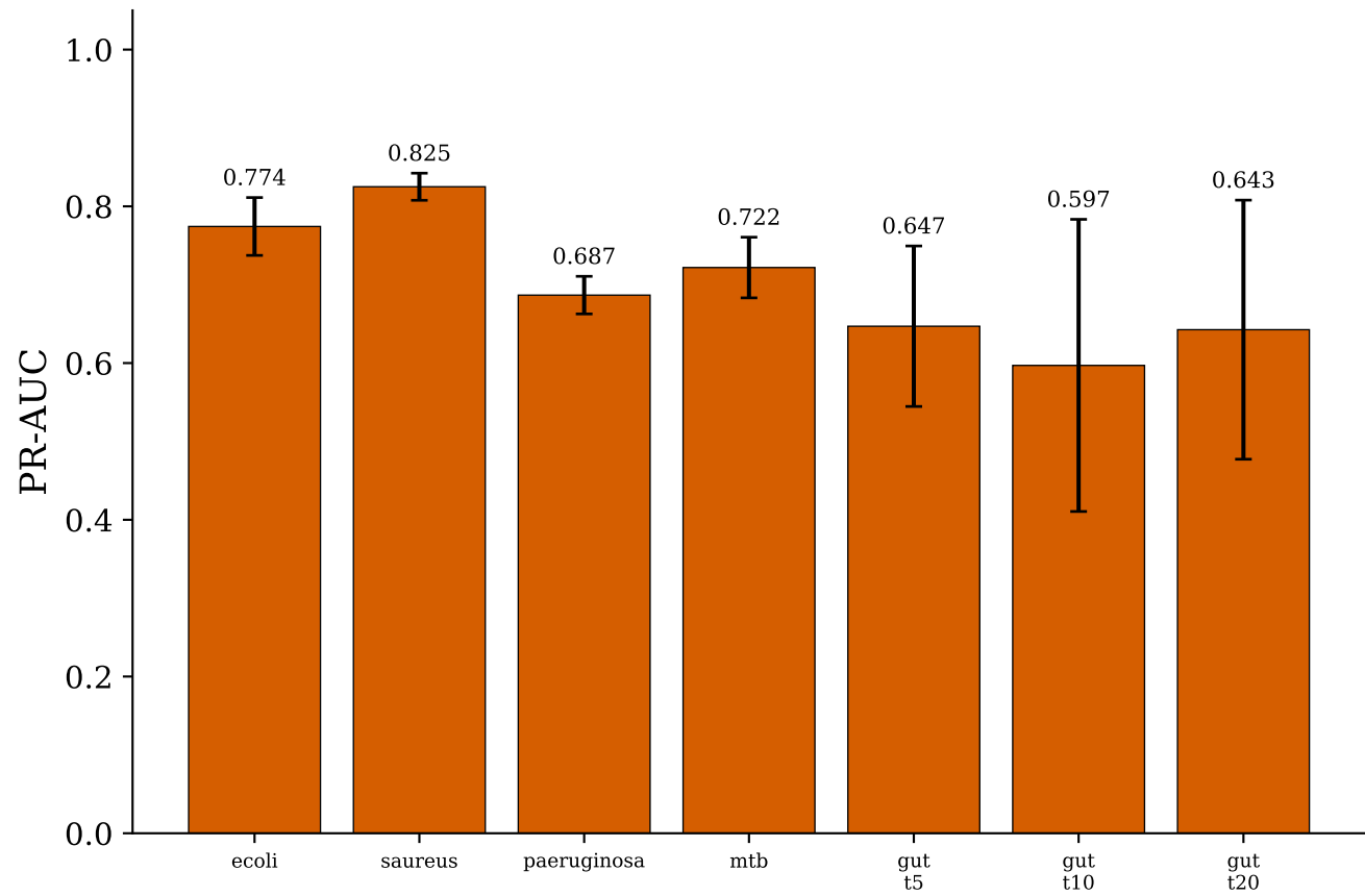
B. D-MPNN PR-AUC (5-fold scaffold CV)
