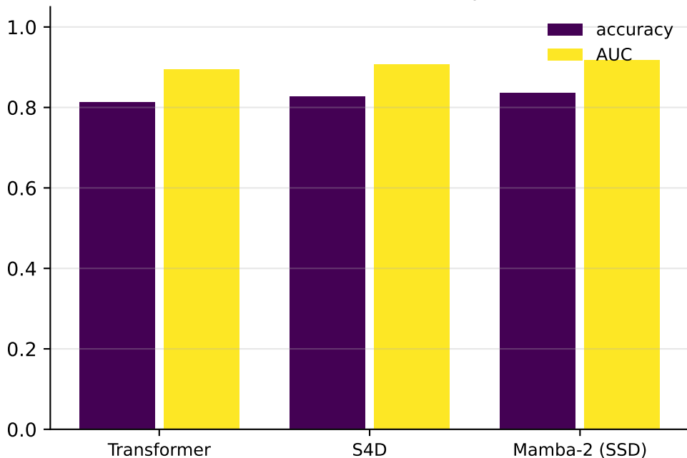
IMDb sentiment (final epoch)
