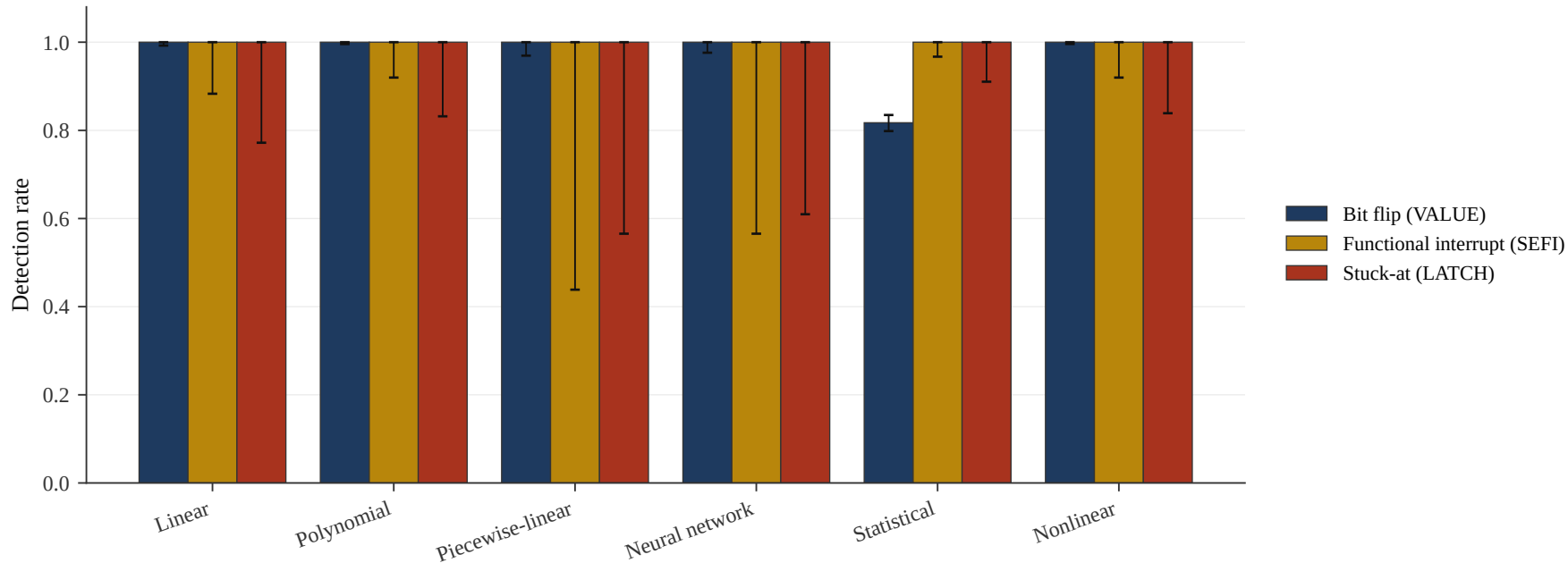
Detection rate per fault class, per frontend (95% Wilson CI)
