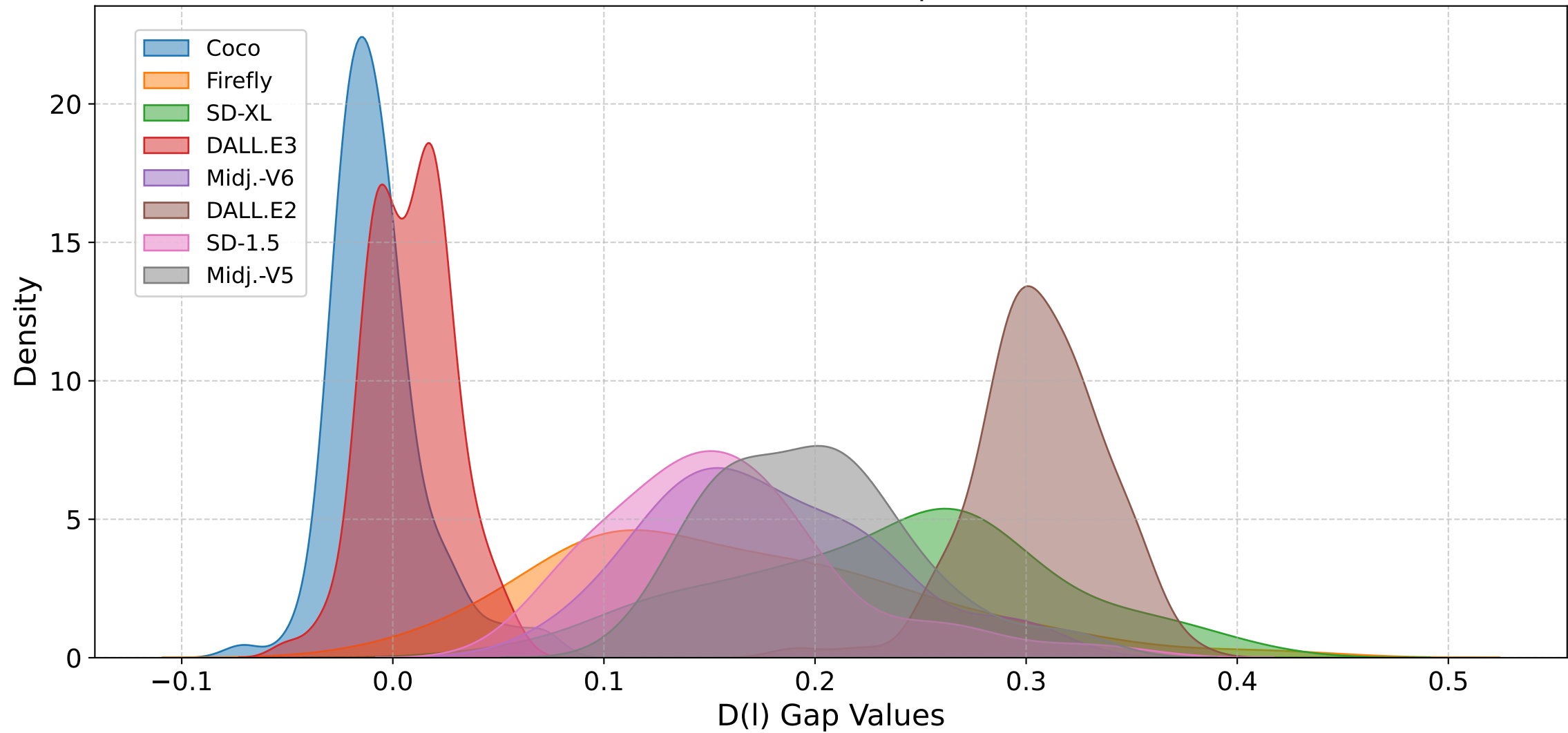
KDE of SReC D(l) Gap Values
