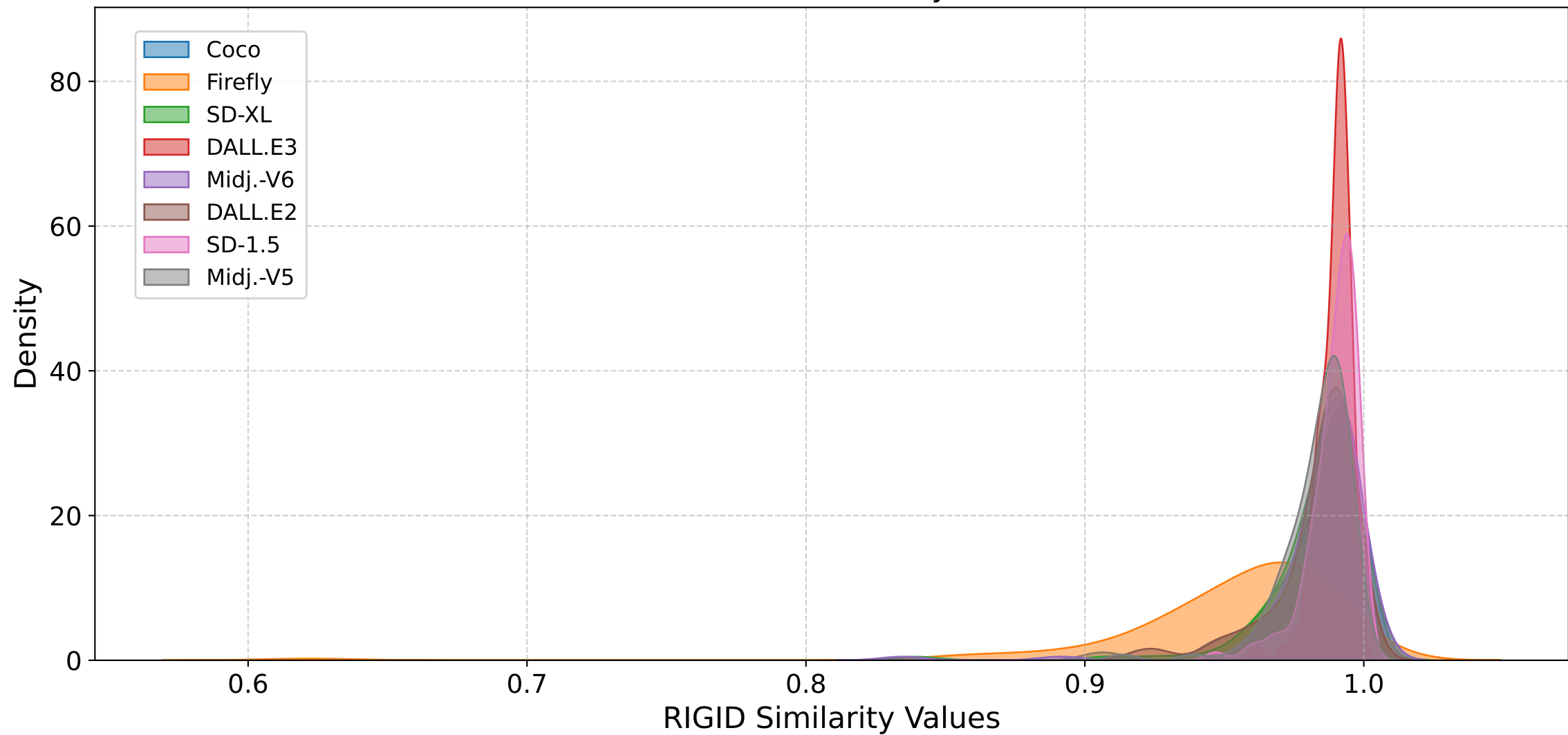
KDE of RIGID Similarity Values
