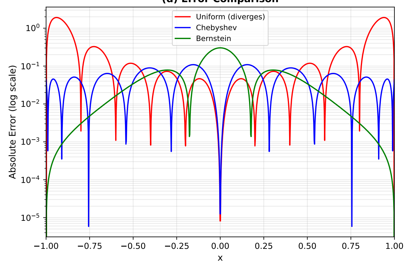
(d) Error Comparison
