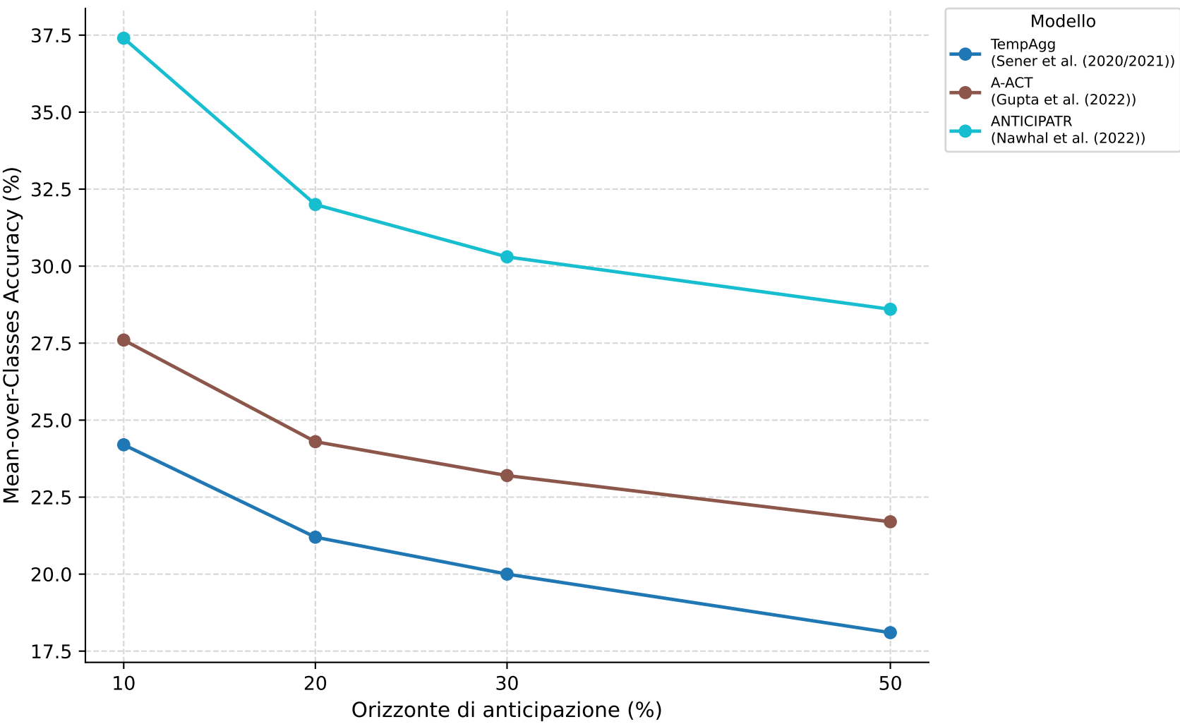
Performance vs. Orizzonte di anticipazione Breakfast Actions · LTA · I3D · Osservazione 20%
