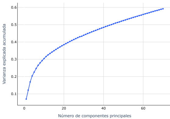
Figura 3. Varianza acumulada en las primeras 70 componentes principales.
