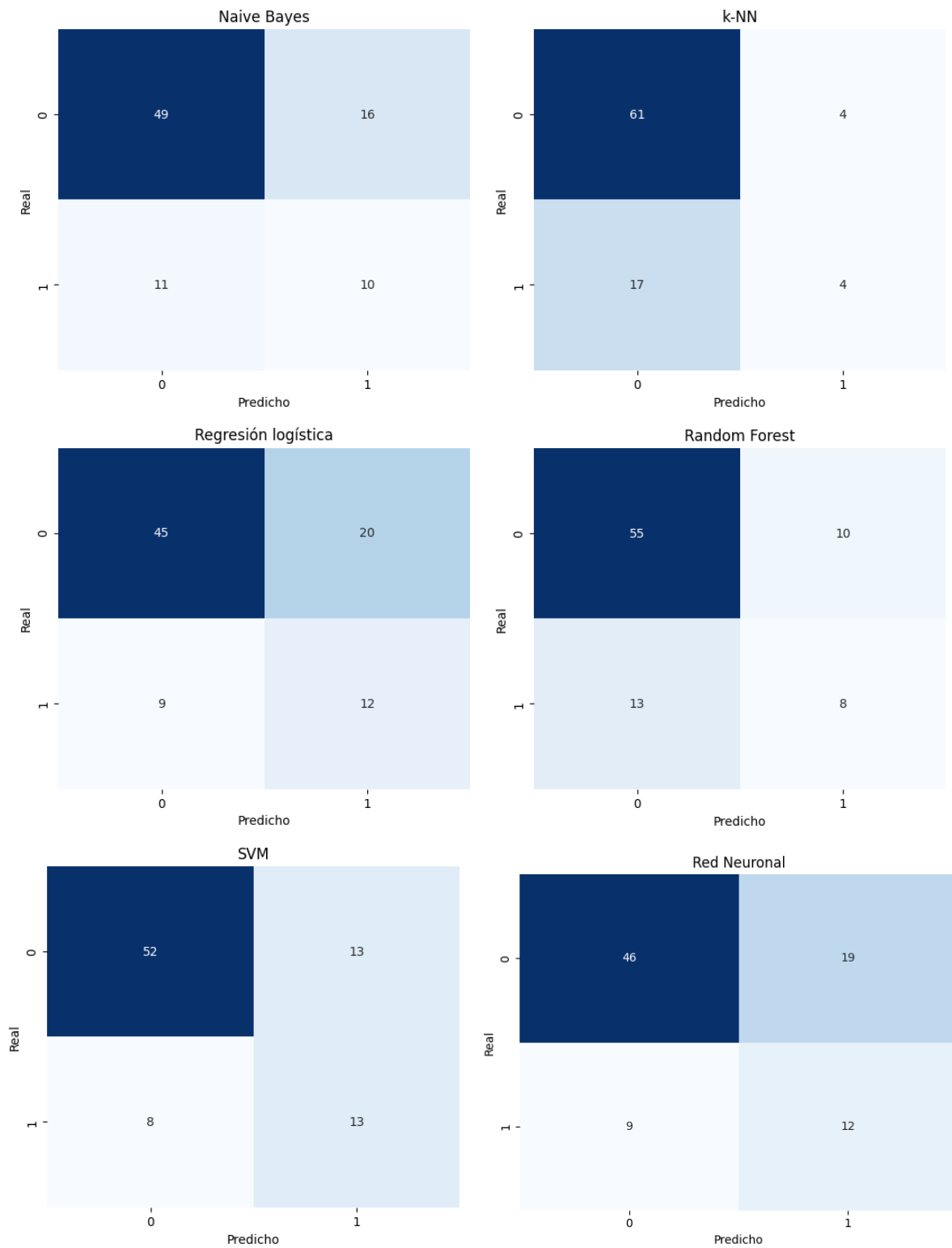
Figura 4. Matrices de confusión de los modelos de clasificación sobre el conjunto de validación.
