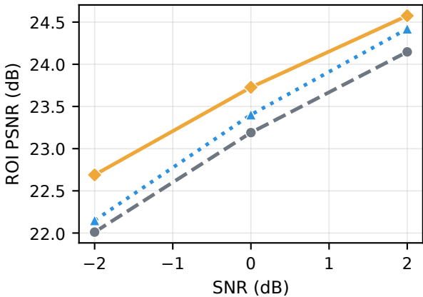
DIV2K Val
