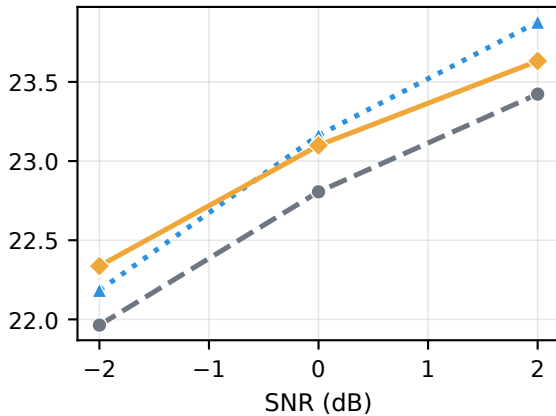
Kodak-24
