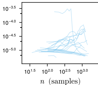
NUTS
