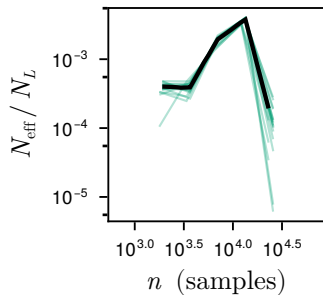
NS
