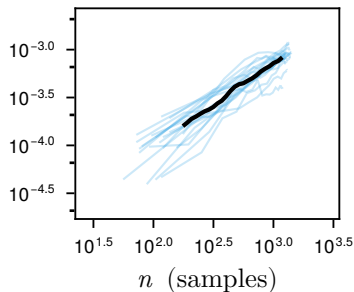
NUTS
