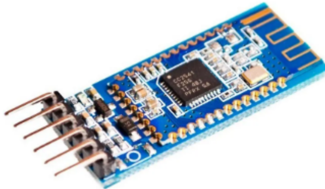
Figura 2.4: módulo HM-10
