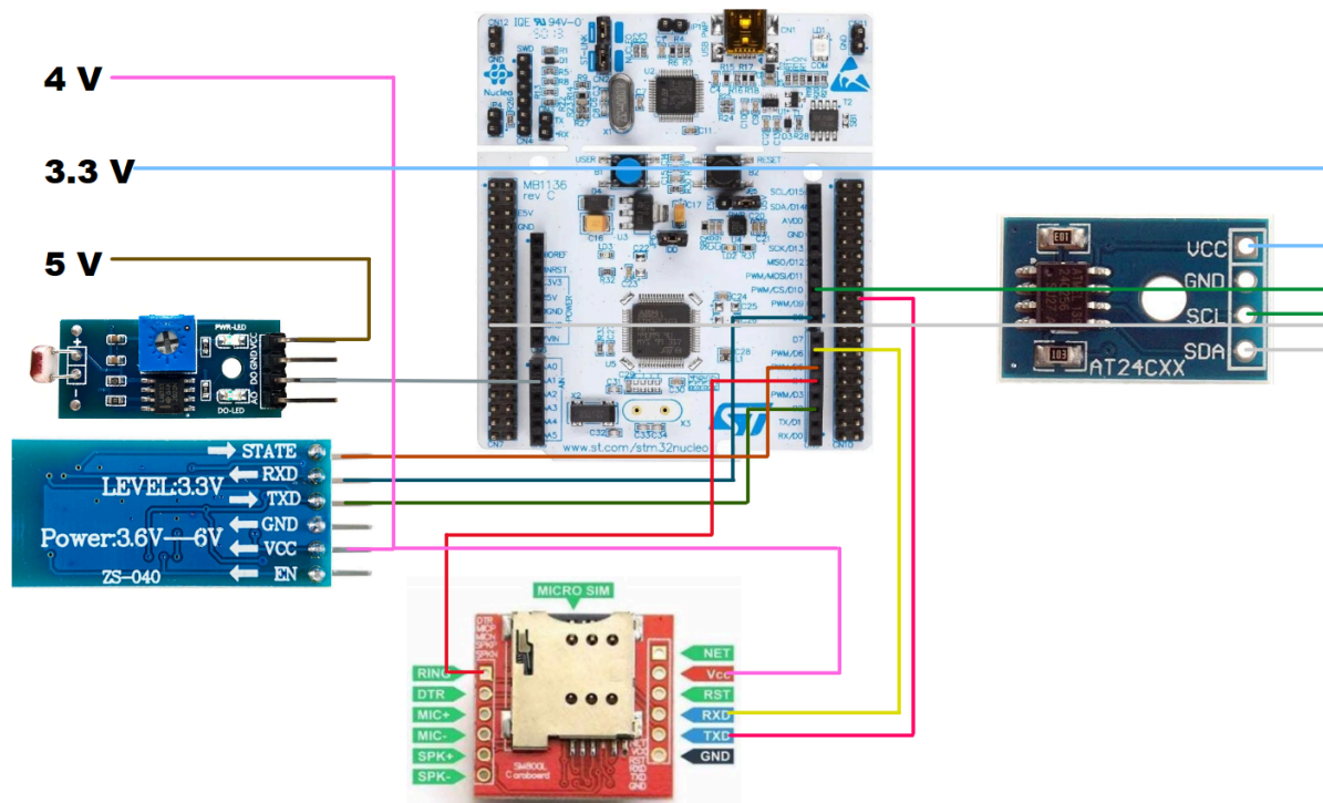
Figura 3.2: Esquema de cableado entre placa y módulos.
