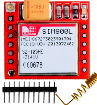
Figura 2.2: módulo GSM.
