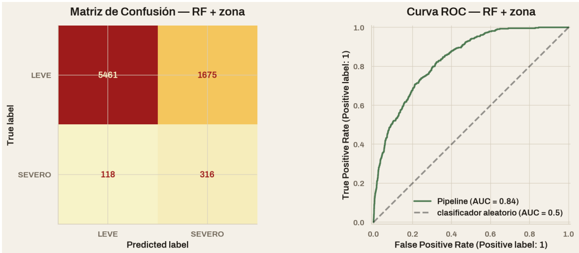
Modelo final Random Forest + zona: matriz de confusión y curva ROC (test 20%, recall SEVERO 0,73).
