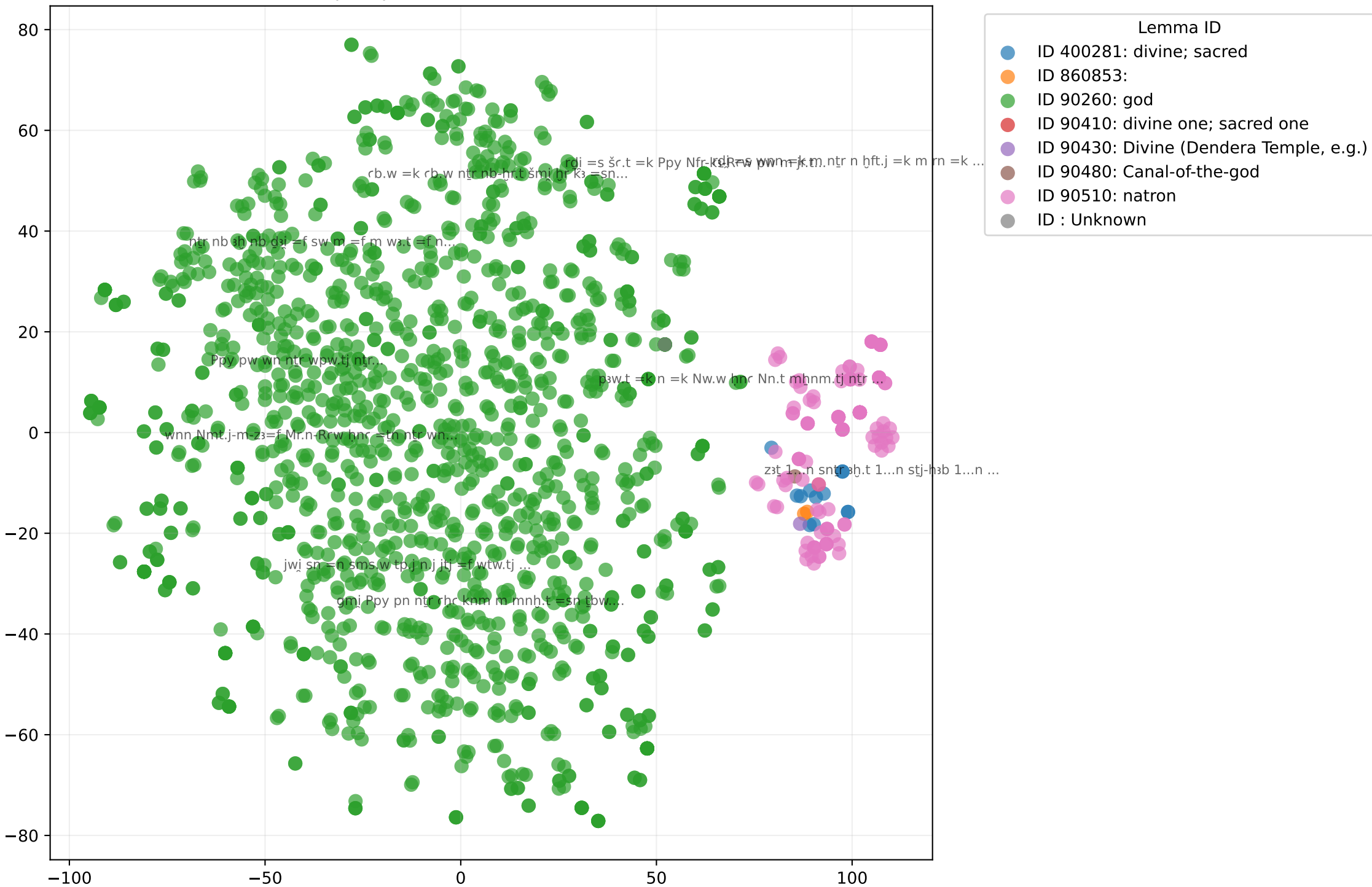
Семантическое пространство контекстов 'ntr' (LaBSE Fine-tuned)
