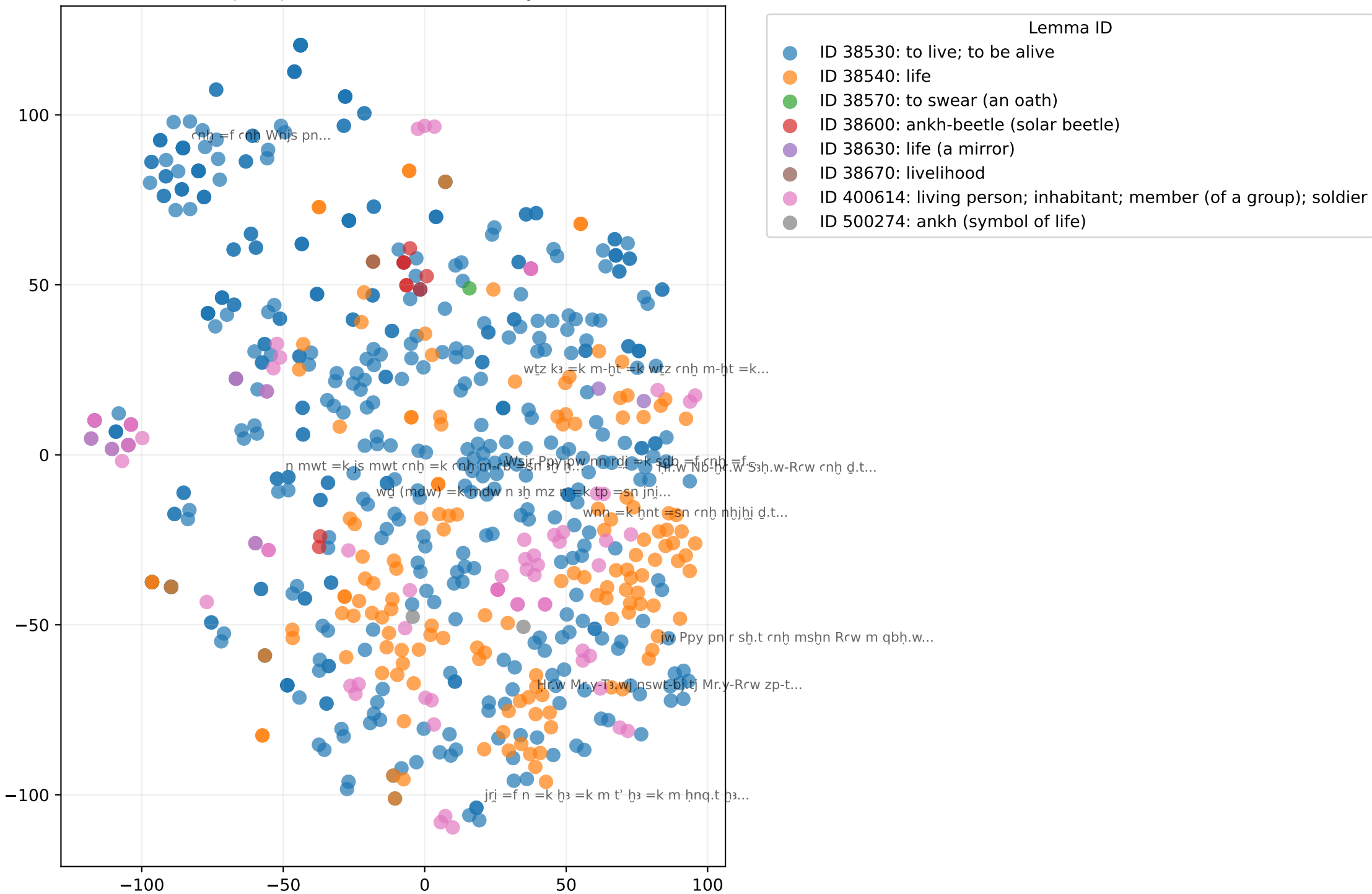
Семантическое пространство контекстов 'rnh' (LaBSE Fine-tuned)
