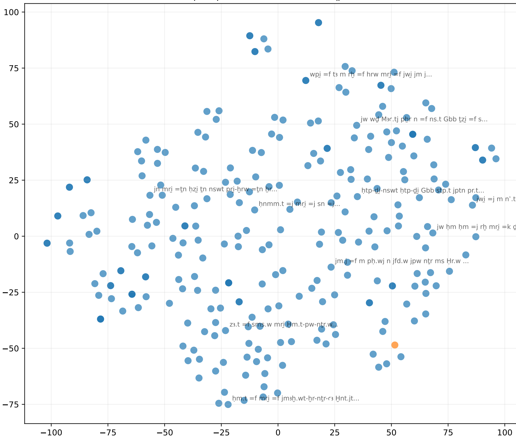
Семантическое пространство контекстов 'mrj' (LaBSE Fine-tuned)
