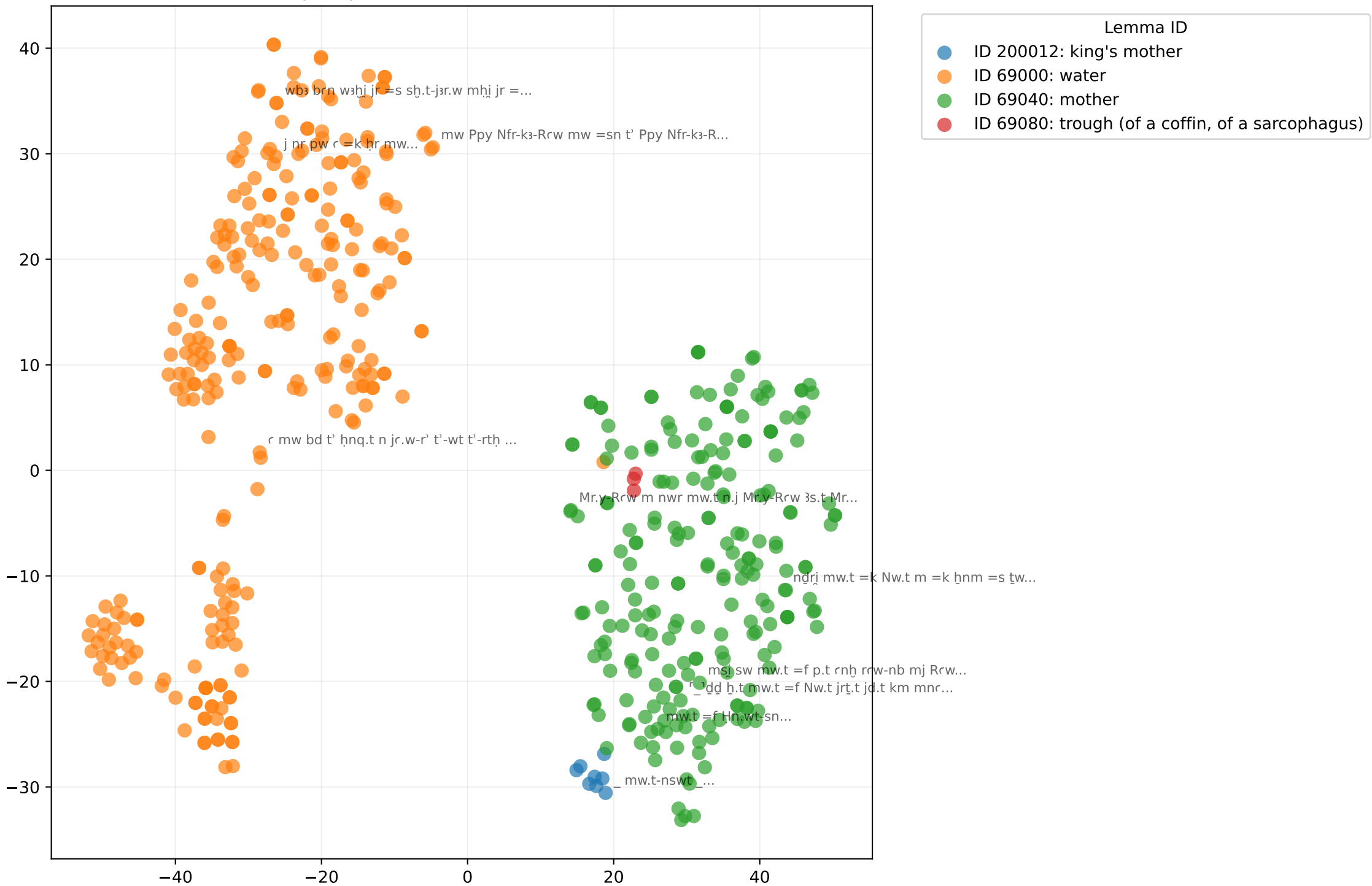
Семантическое пространство контекстов 'mw' (LaBSE Fine-tuned)
