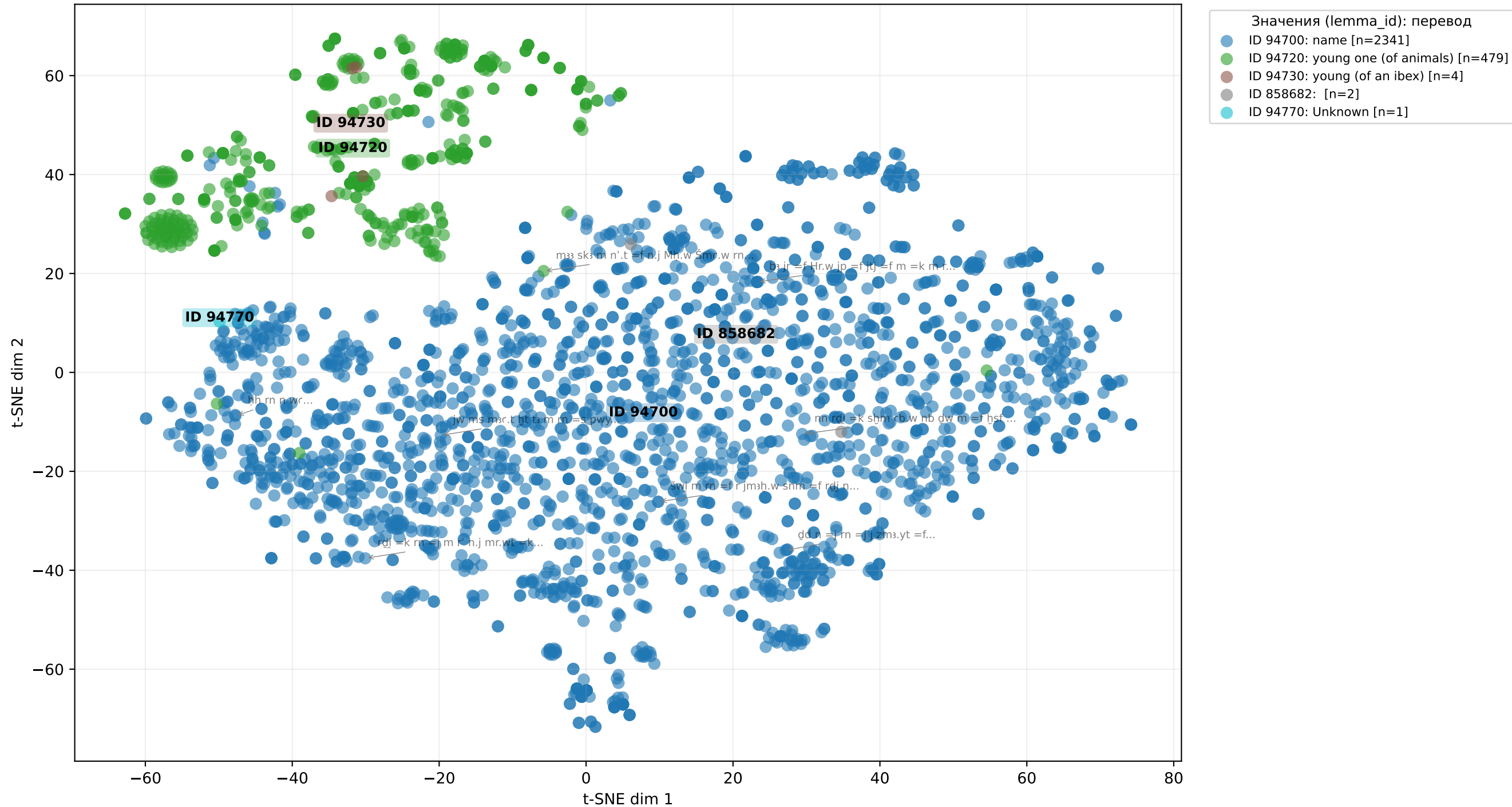
WSI: «rn» — 2827 контекстов, 5 значений ARI=0.239, Silhouette=-0.211 | стратегия: plain | SONAR curriculum
