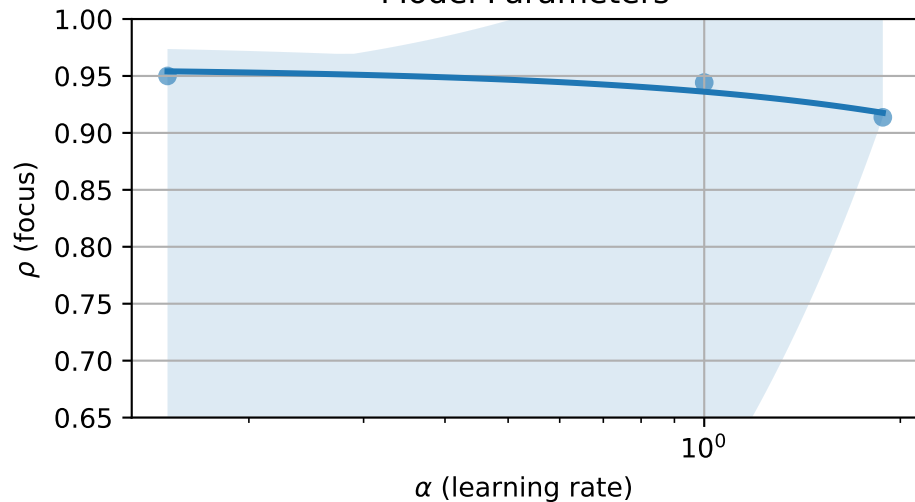
Model Parameters
