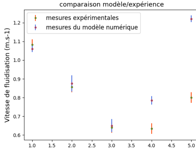
FIGURE 16 – Comparaison des vitesses de fluidisation V_{mf} obtenues expérimentalement (barres d'erreur oranges) et par le modèle numérique DEM (barres d'erreur bleues) pour les cinq milieux granulaires étudiés (1 : sable fin, 2 : sel, 3 : graines de chia, 4 : quinoa, 5 : lentilles). Les barres d'erreur représentent l'écart-type des mesures répétées.
