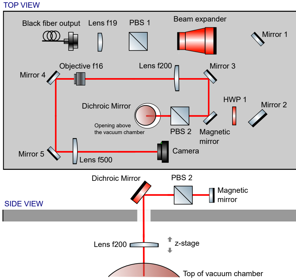
Figure 2.18: Questa è un'immagine vettoriale caricata da un PDF. MI sa che l'AOM va ruotato
