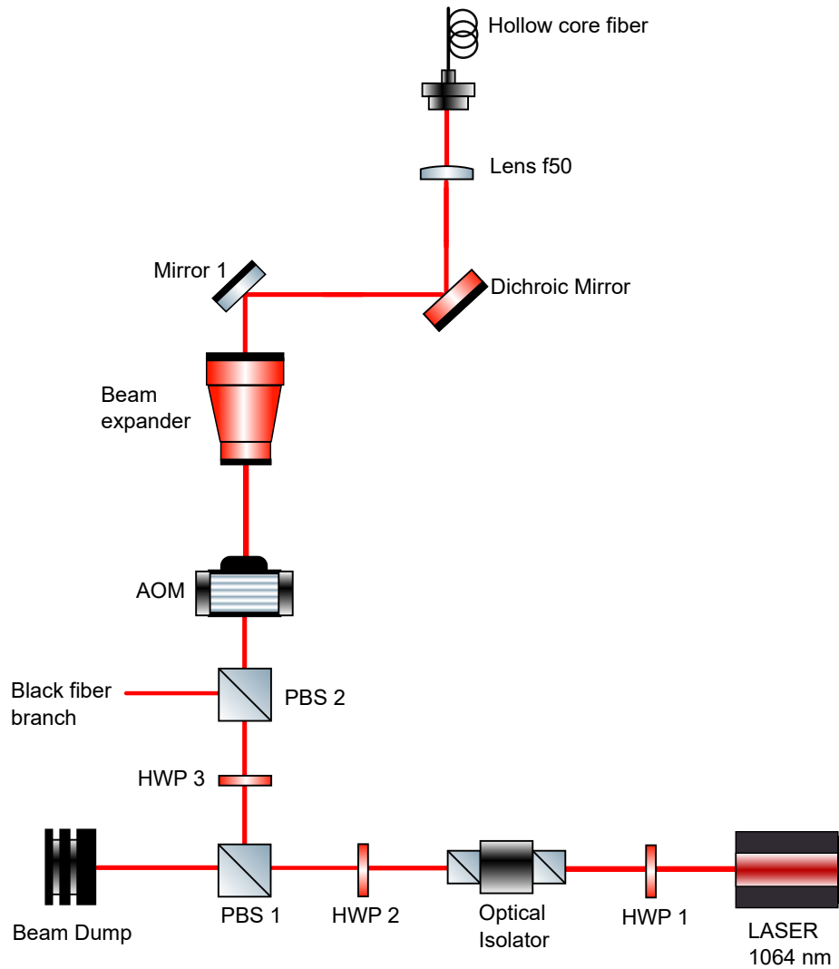
Figure 2.9: Questa è un'immagine vettoriale caricata da un PDF. MI sa che l'AOM va ruotato
