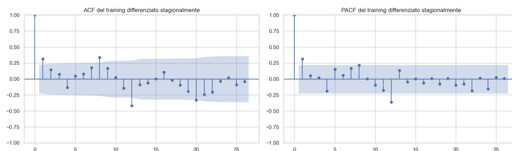
Figura 5.5: ACF e PACF del training differenziato stagionalmente.
