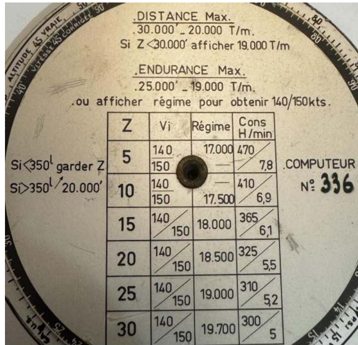
Face « 336 » — table régime / consommation et règle à calcul circulaire.
