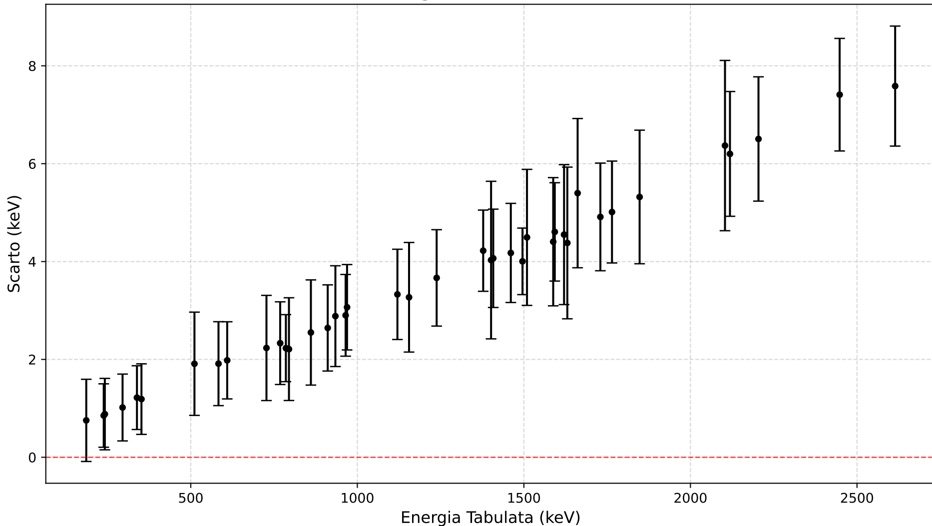
Scarto Energie: Misurate vs Tabulate
