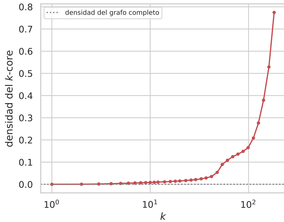
Densidad interna del k -core
