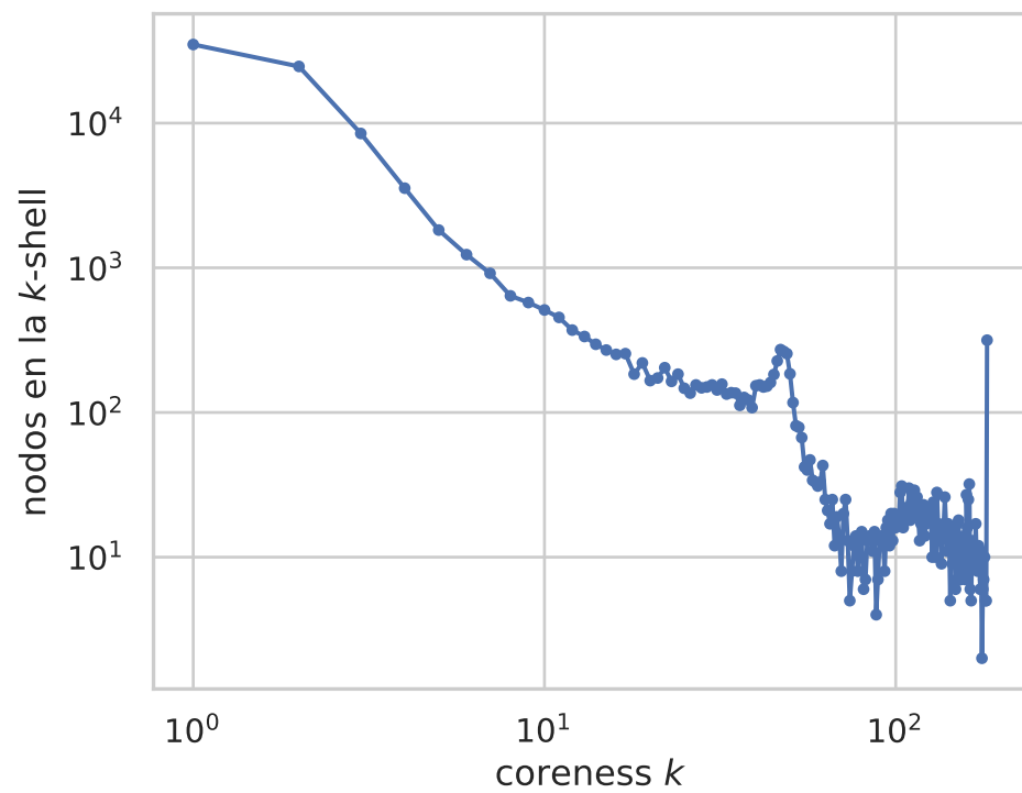
Tamaño de las k -shells
