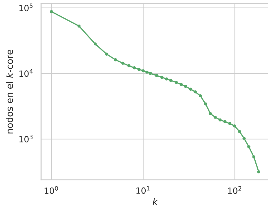
Tamaño del k -core
