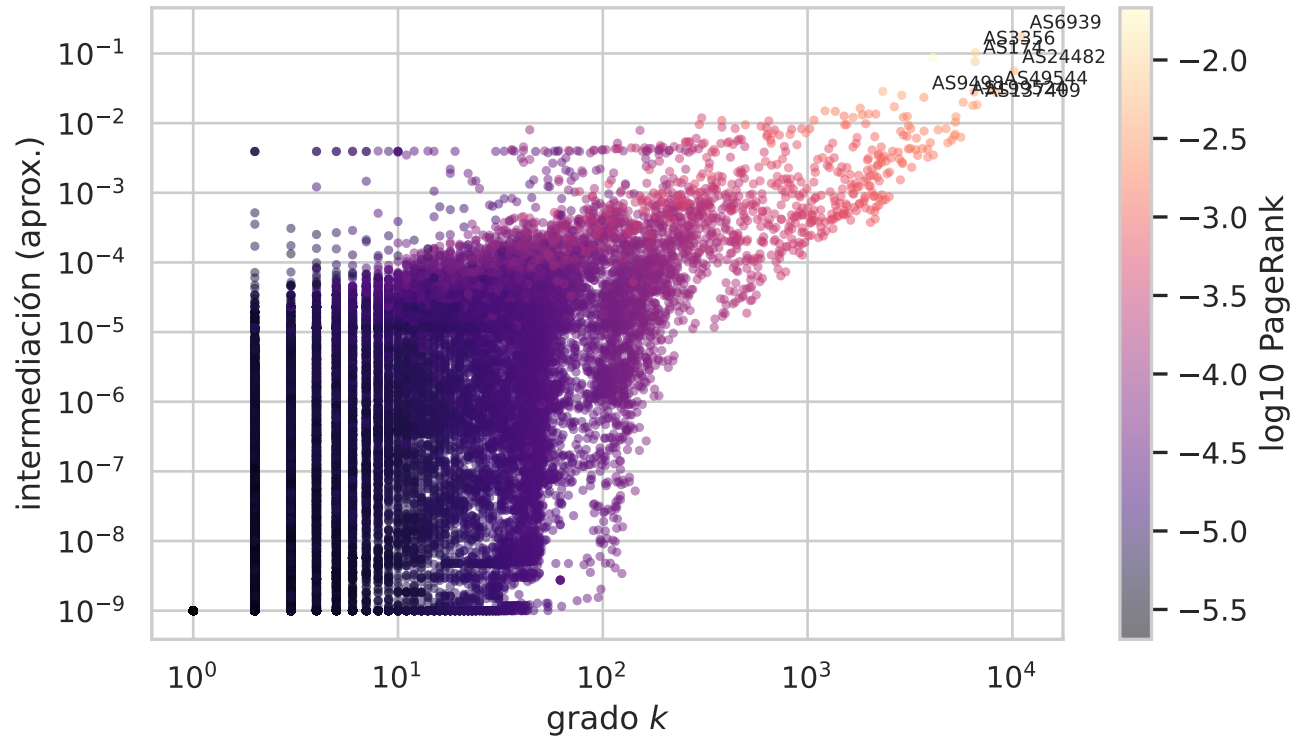
Grado vs intermediación (color = \log_{10} PageRank)
