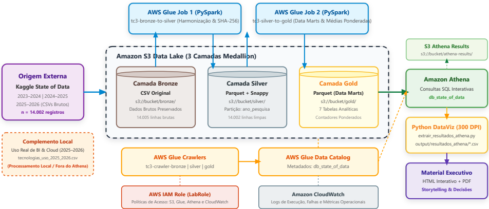
Arquitetura da Plataforma de Dados — Data Lakehouse em 3 Camadas Medallion na Amazon S3 com AWS Glue, PySpark e Amazon Athena
