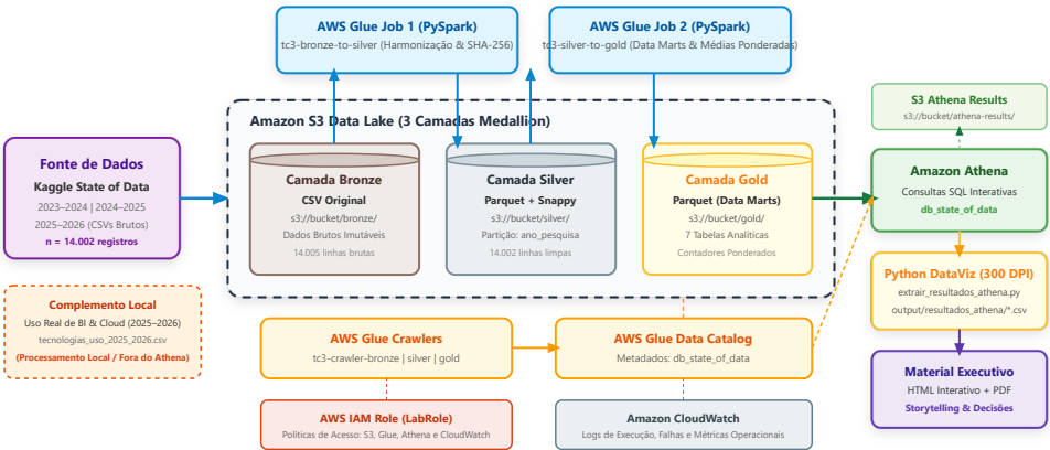
Arquitetura Oficial — Tech Challenge Fase 3 (Data Lakehouse em 3 Camadas Medallion no Amazon S3 com AWS Glue, PySpark e Athena)
