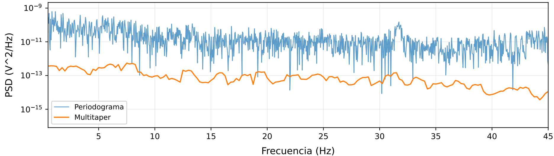
Periodograma vs multitaper por estado: Ojos cerrados
