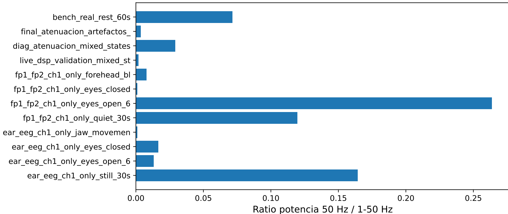
Comparación de ratio de ruido 50 Hz
