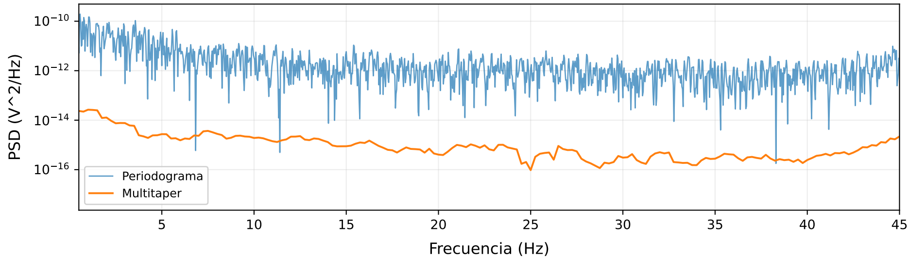
Periodograma vs multitaper por estado: Ojos abiertos
