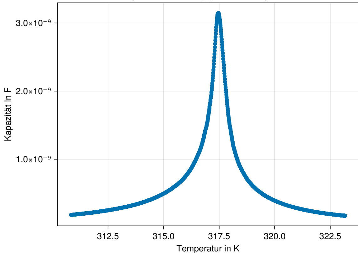
Kapazität in Abhängigkeit der Temperatur
