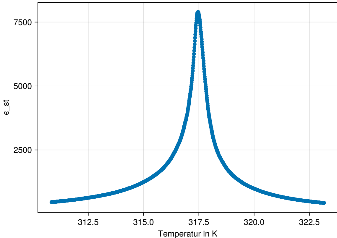
\epsilon_{st} in Abhängigkeit der Temperatur
