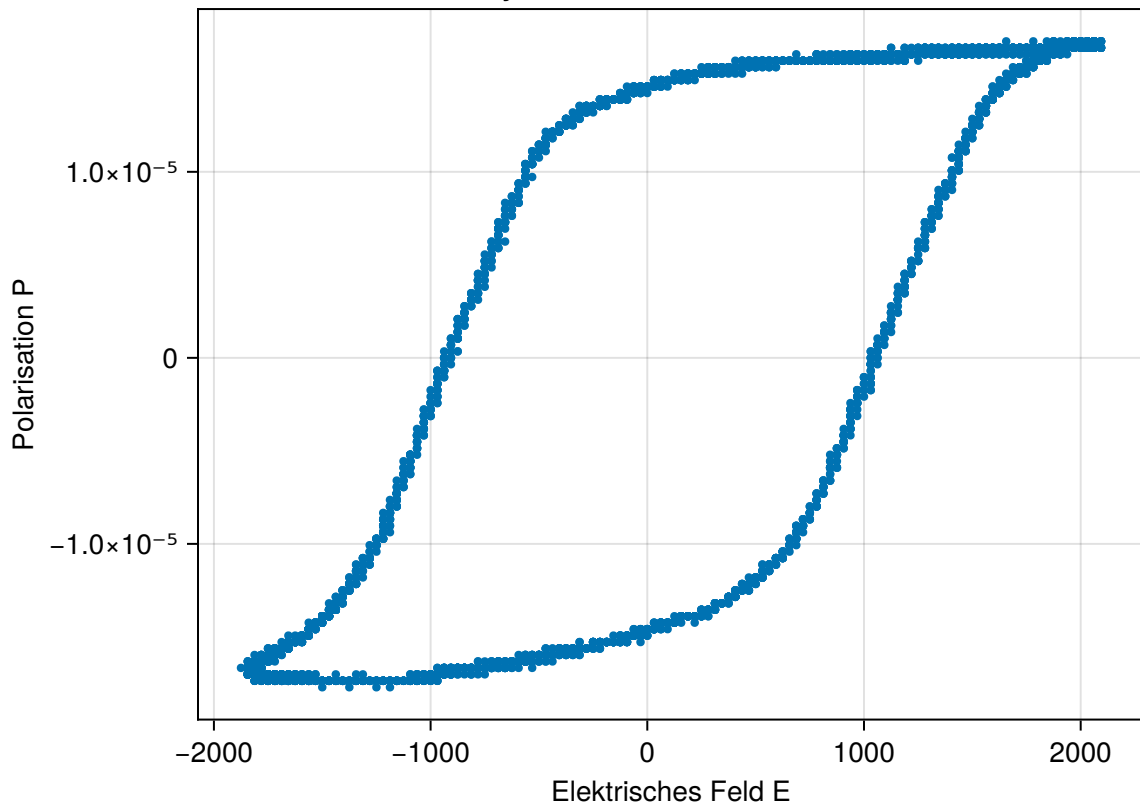
Hysteresese bei 4V und 115 Hz
